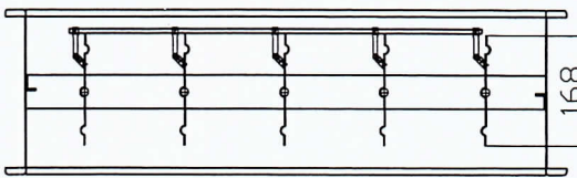
A-A剖面图叶片打开状态
