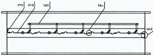
A-A剖面图叶片关闭状态
