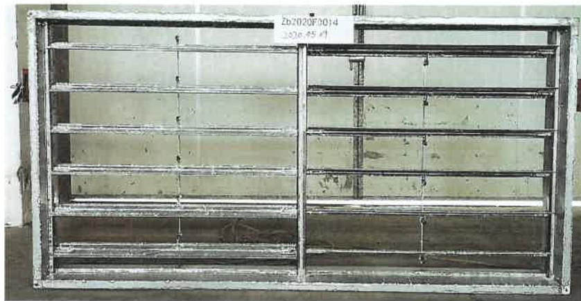
照片 1 耐腐蚀性试验后试件叶片打开状态
